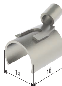
081154-_2 Crimp Type Cable Lug
